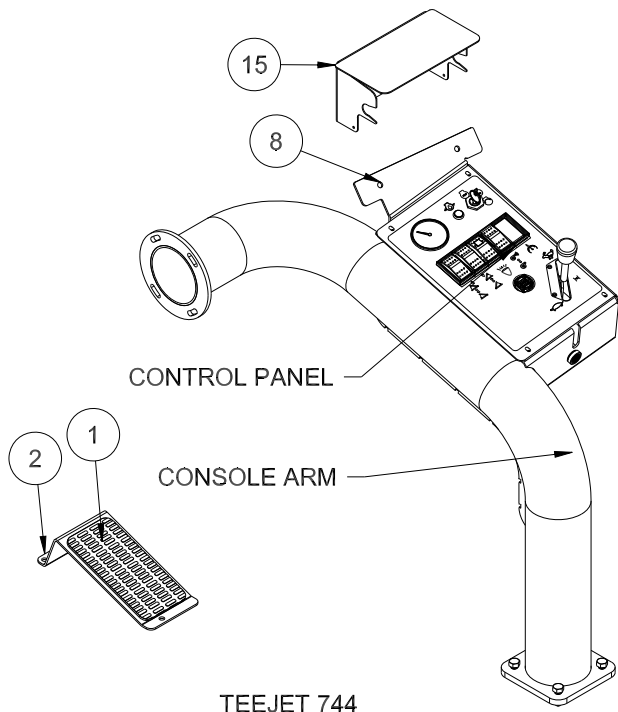
TEEJET 744
