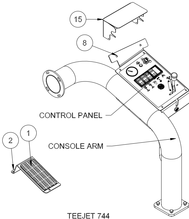
TEEJET 744
