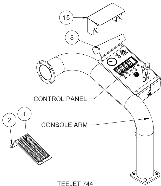
TEEJET 744
