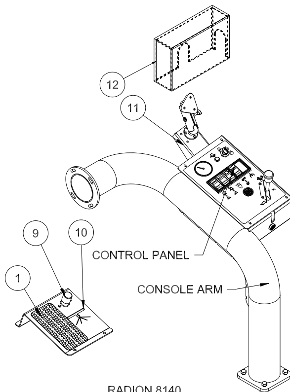
RADION 8140
